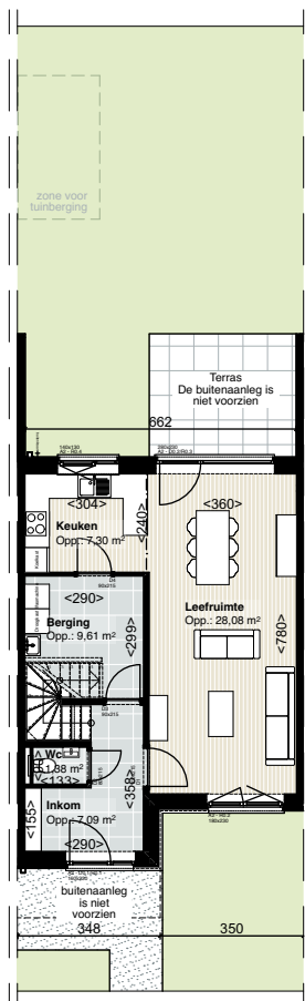
GRONDPLAN GELIJKVLOERS SCHAAL 1/200
