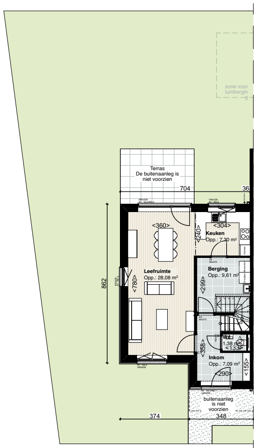
GRONDPLAN GELIJKVLOERS SCHAAL 1/200
