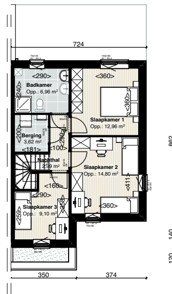
GRONDPLAN VERDIEPING SCHAAL 1/200
