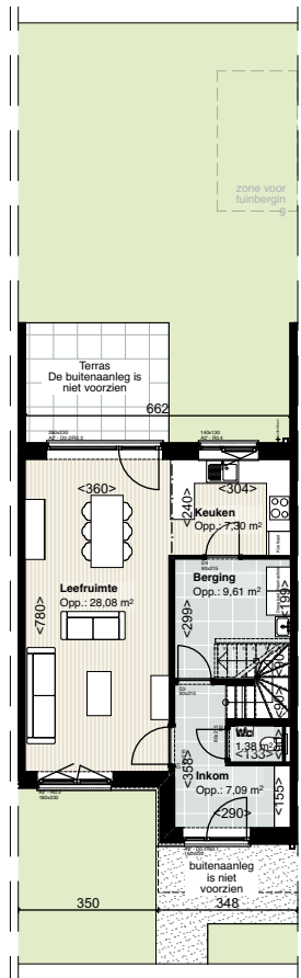
GRONDPLAN GELIJKVLOERS SCHAAL 1/200
