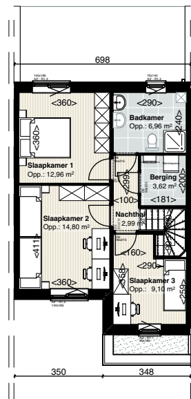
GRONDPLAN VERDIEPING SCHAAL 1/200
