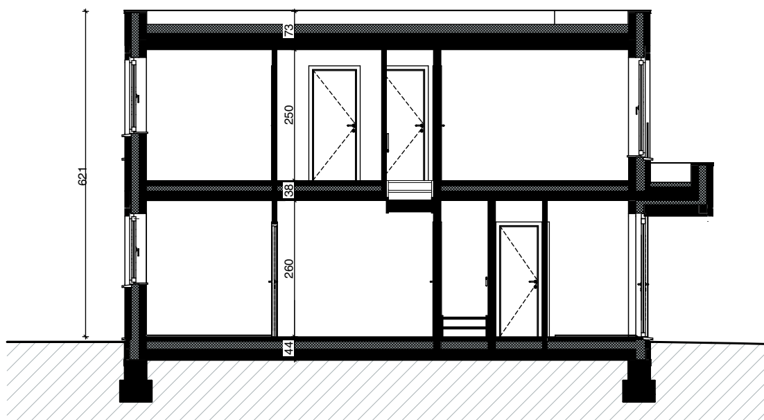
DOORSNEDE SCHAAL 1/100
