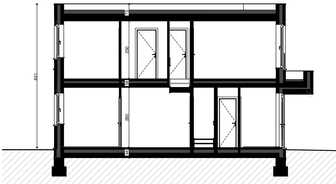
DOORSNEDE SCHAAL 1/200
