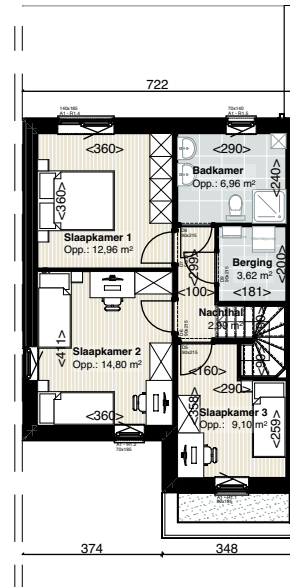
GRONDPLAN VERDIEPING SCHAAL 1/200
