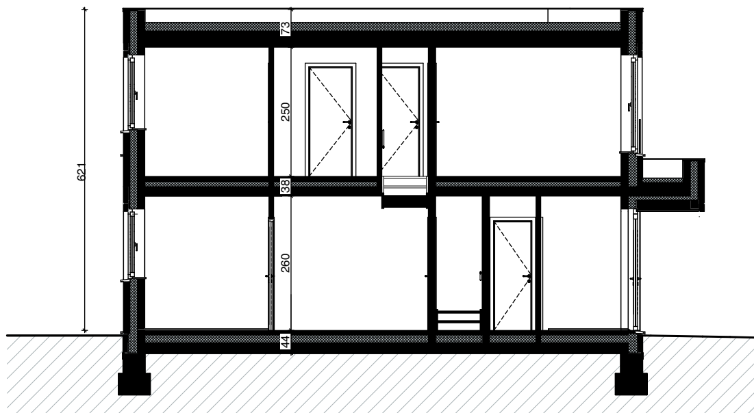
DOORSNEDE SCHAAL 1/100
