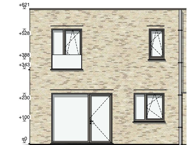
ACHTERGEVEL SCHAAL 1/200
