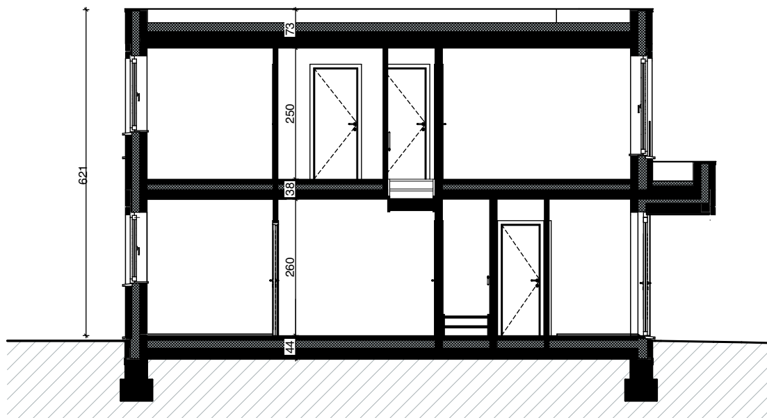
DOORSNEDE SCHAAL 1/100
