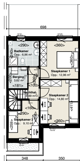
GRONDPLAN VERDIEPING SCHAAL 1/200
