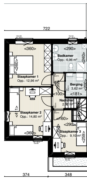
GRONDPLAN VERDIEPING SCHAAL 1/200
