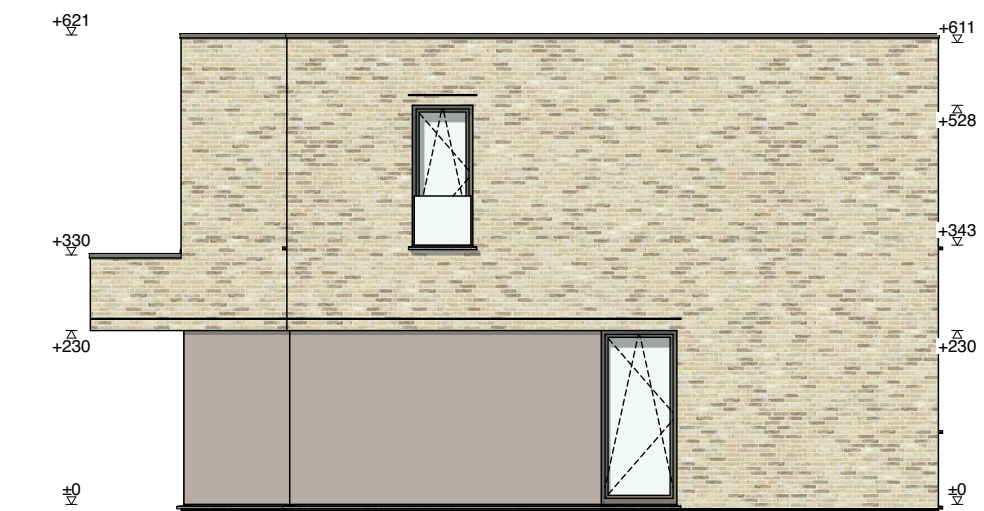
RECHTERGEVEL SCHAAL 1/200
